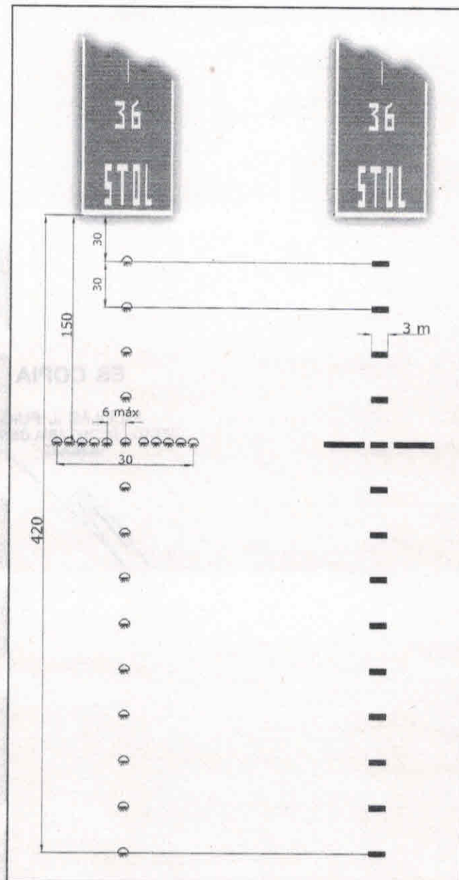
Figura E-5 Sistema de iluminación de aproximación
