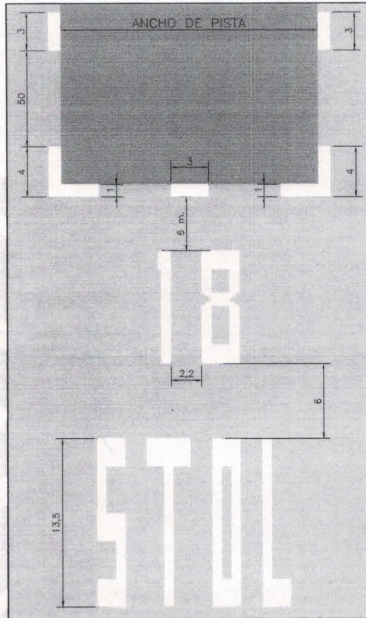
Figura E-2 Señal de umbral STOL en pistas no pavimentadas
