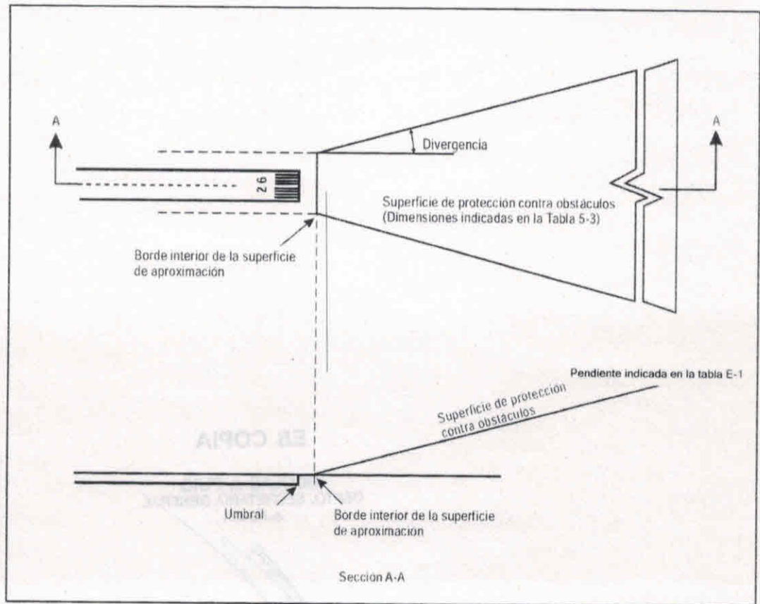
Figura E-7 Superficie de protección contra obstáculos para los Sistemas Visuales Indicadores de Pendiente de Aproximación
