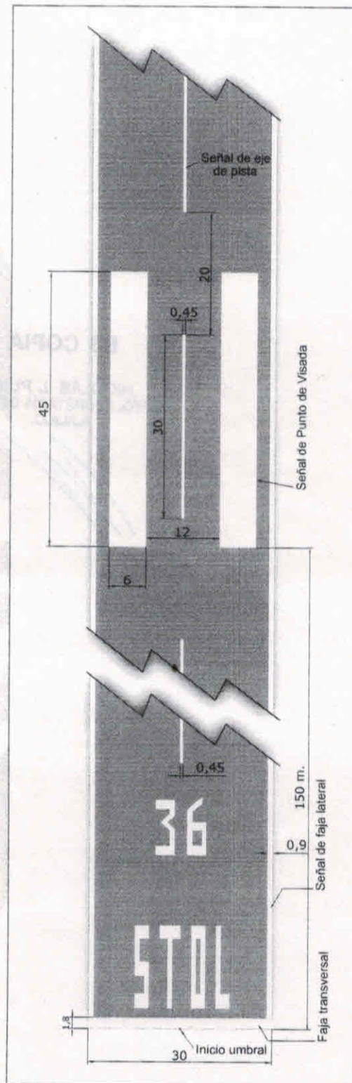
Figura E-4 Señal de Punto de Visada
