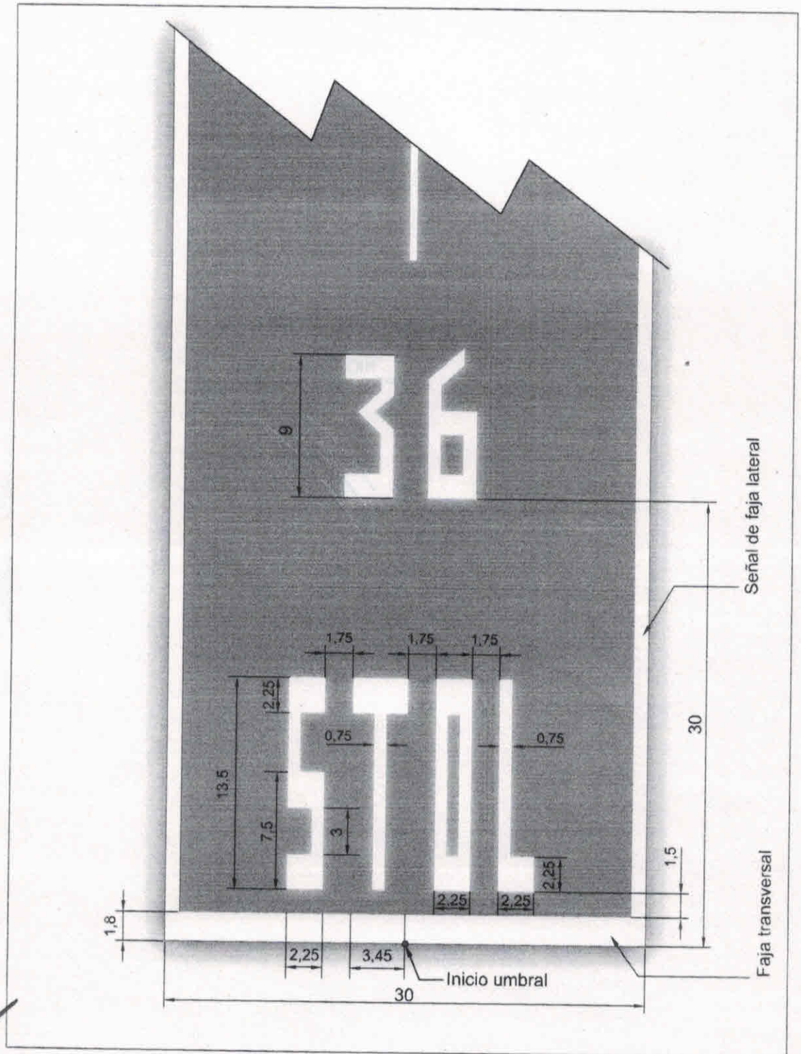
Figura E-3 Señal de umbral STOL en pistas pavimentadas
