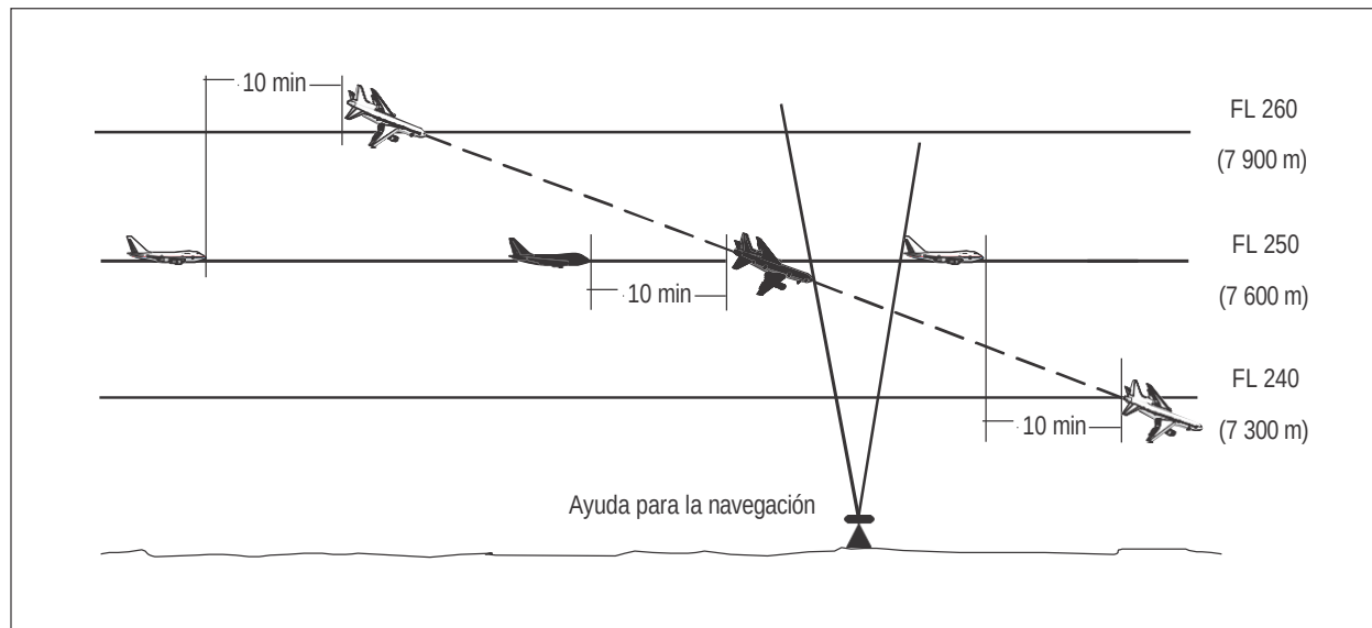
Figura 5-20B. Separación de 10 minutos entre aeronaves que descienden y por derrotas que se cruzan [véase 5.4.2.2.2 b)]
