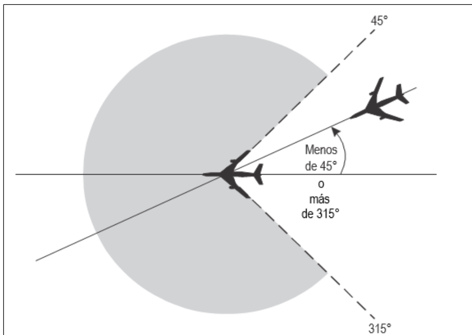
Figura 5-7. Aeronaves por la misma derrota [véase 5.4.2.1.5 a)]
