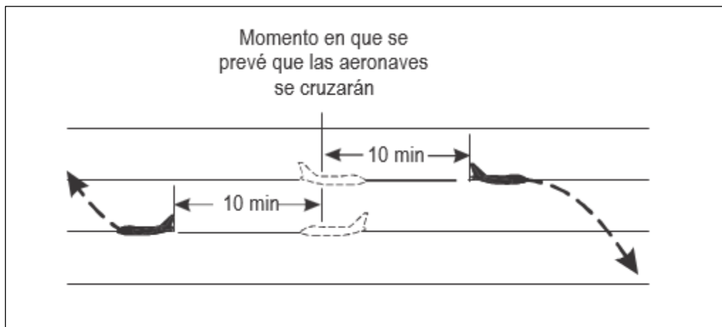
Figura 5-21. Separación de 10 minutos entre aeronaves por derrotas opuestas (véase 5.4.2.2.3)
