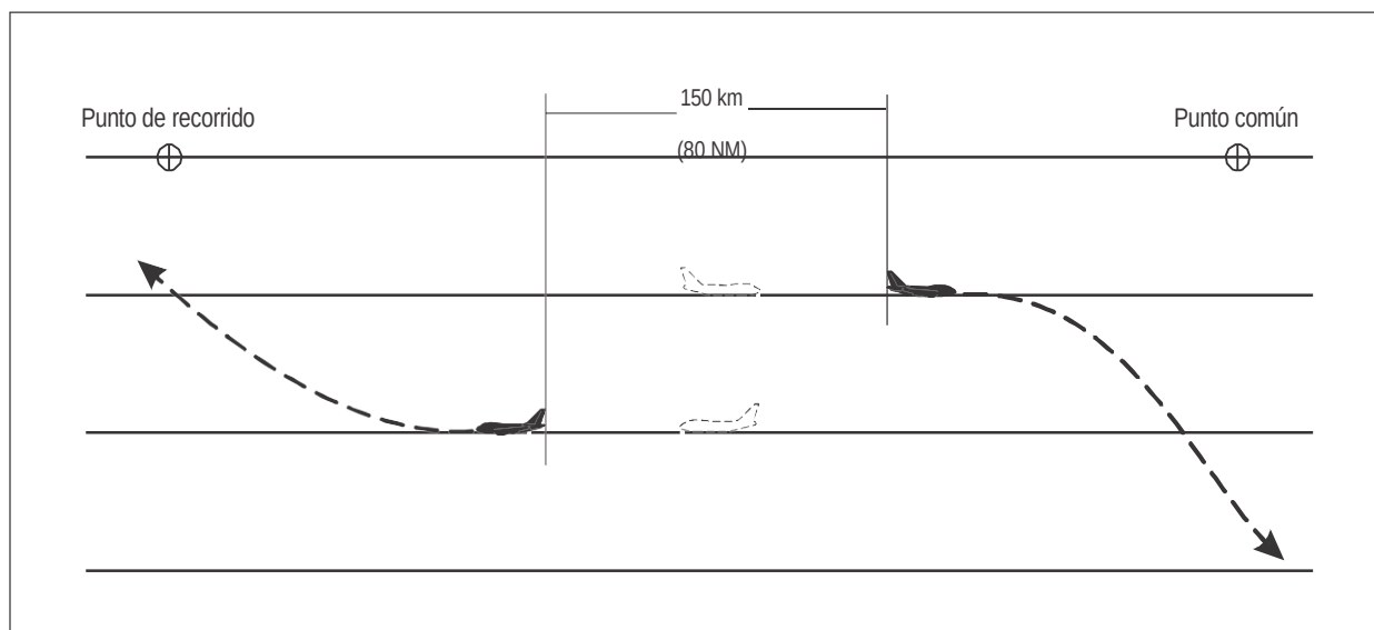
Figura 5-28. Separación de 150 km (80 NM) basada en RNAV entre aeronaves por derrotas opuestas (véase 5.4.2.5.7)
