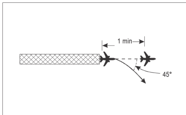
Figura 5-37. Un minuto de separación entre aeronaves que salen y siguen derrotas divergentes por lo menos en 45^\circ (véase 5.6.1)
