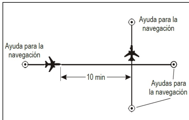
Figura 5-15. Separación de 10 minutos entre aeronaves por derrota que se cruzan y al mismo nivel [véase 5.4.2.2.1.2 b)]
