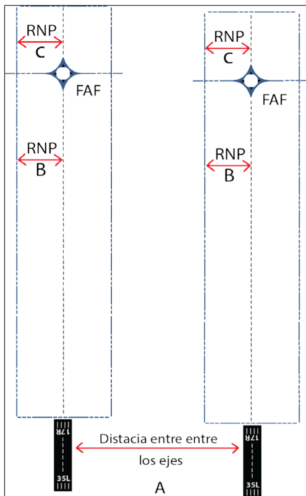
Figura 6-2 — Valor RNP y distancia entre los ejes de las pistas
