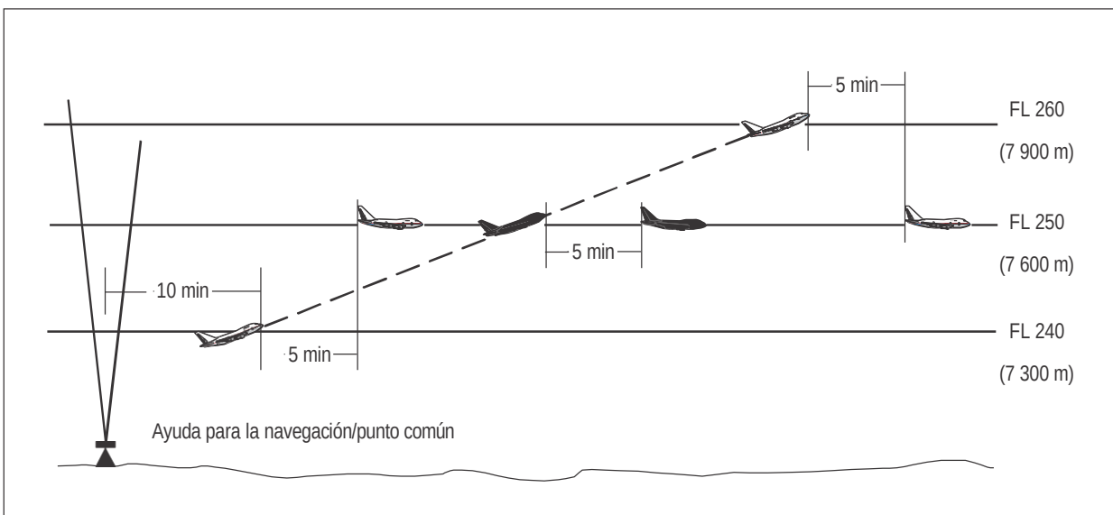
Figura 5-18A. Separación de 5 minutos entre aeronaves que ascienden y por la misma derrota [véase 5.4.2.2.1 c) 2)]
