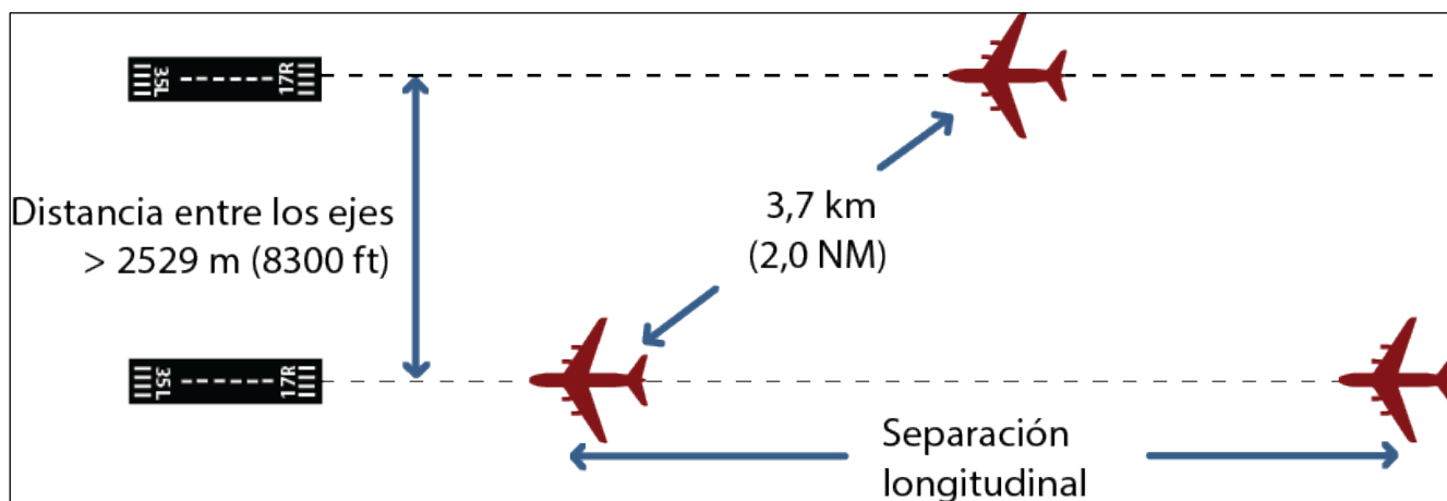
Figura 6-3. Separación diagonal para una distancia entre ejes mayor que 2 529 m (8 300 ft)
