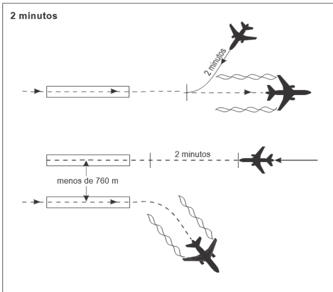
Figura 5-46. Separación de 2 minutos por estela turbulenta para aterrizajes en sentidos opuestos [véase 5.8.5 b)]
