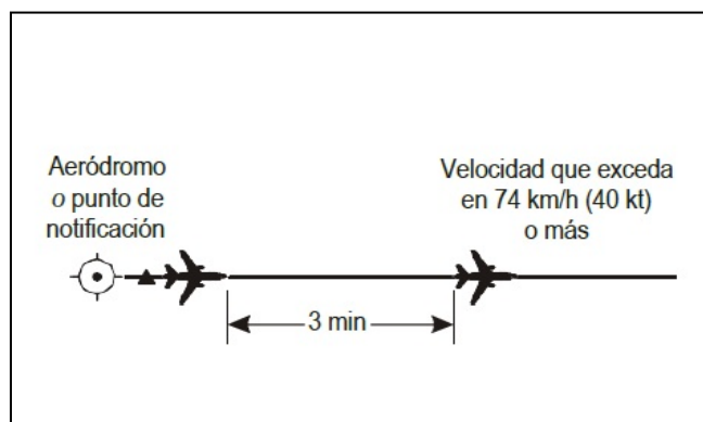
Figura 5-13. Separación de 3 minutos entre aeronaves por la misma derrota y el mismo nivel [véase 5.4.2.2.1.1 d)]
