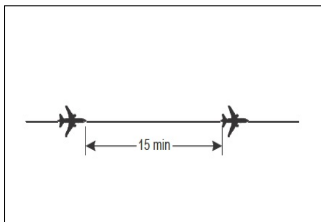
Figura 5-10. Separación de 15 minutos entre aeronaves por la misma derrota y el mismo nivel [véase 5.4.2.2.1.1 a)]
