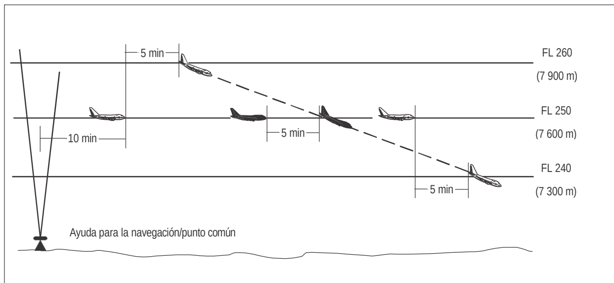
Figura 5-18B. Separación de 5 minutos entre aeronaves que descienden y por la misma derrota [véase 5.4.2.2.2.1 c) 2)]
