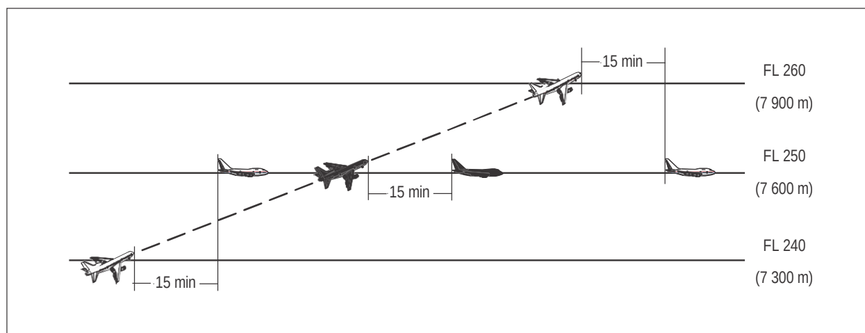
Figura 5-19A. Separación de 15 minutos entre aeronaves que ascienden y por derrota que se cruzan [véase 5.4.2.2.2.2 a) ]
