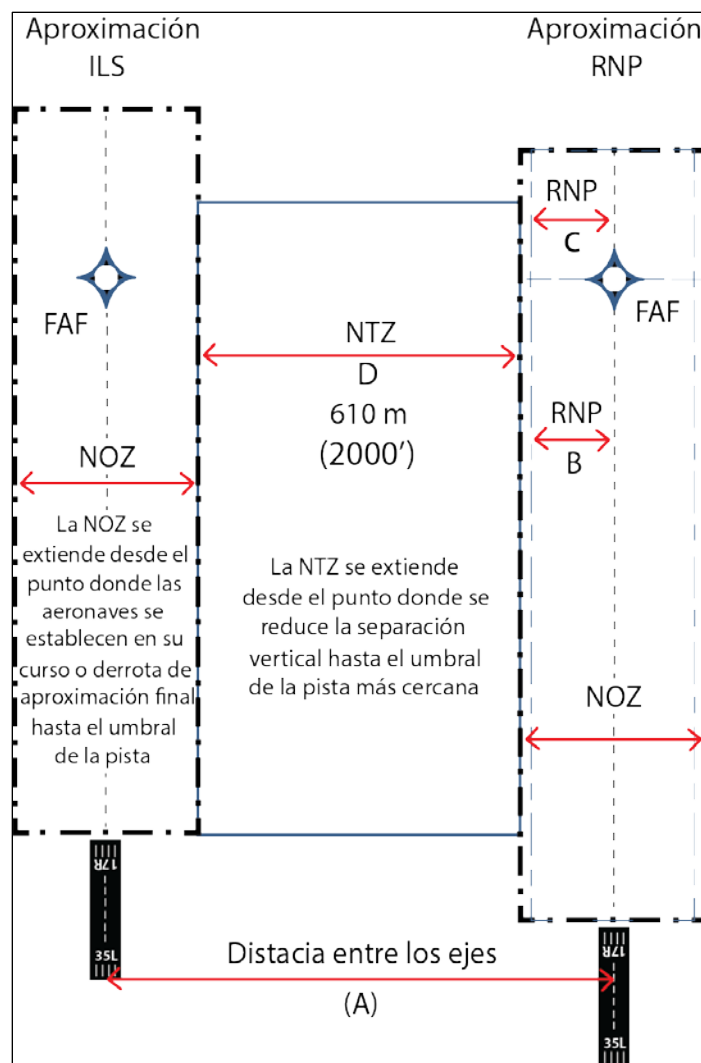
Figura 6-1 Distancia entre los ejes de las pistas, NTZ y NOZ
