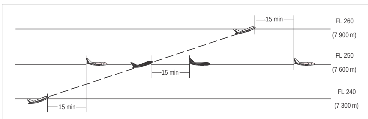
Figura 5-16A. Separación de 15 minutos entre aeronaves que ascienden y por la misma derrota [véase 5.4.2.2.2.1 a)]
