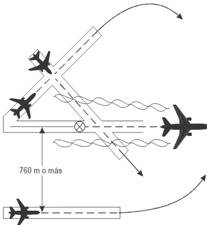
Figura 5-43. Separación de 2 minutos por estela turbulenta para aeronaves que se cruzan [véase 5.8.3.1 c) y d)]
