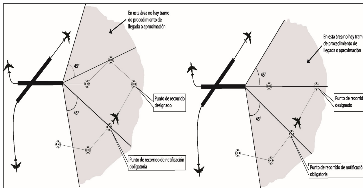
Figura 5-41. Área de protección de llegada
