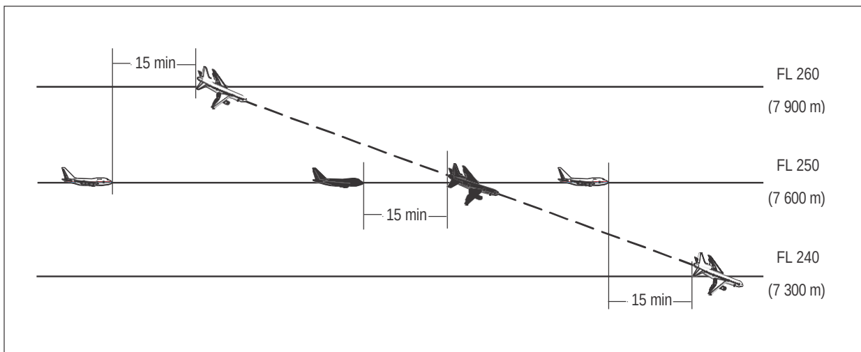
Figura 5-19B. Separación de 15 minutos entre aeronaves que descienden y por derrotas que se cruzan [véase 5.4.2.2.2 a) ]
