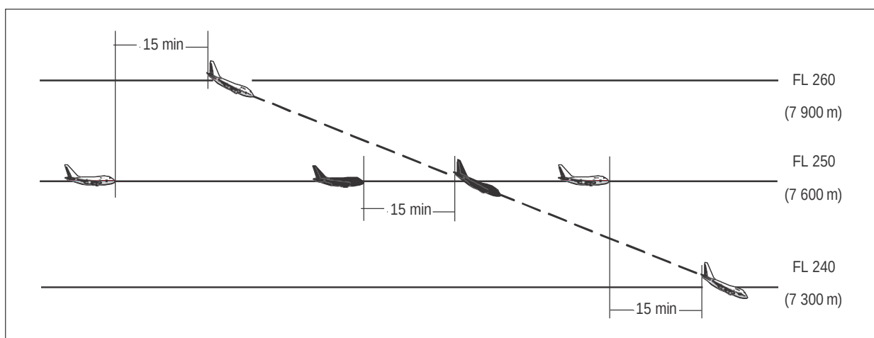
Figura 5-16B. Separación de 15 minutos entre aeronaves que descienden y por la misma derrota [véase 5.4.2.2.2.1a)]
