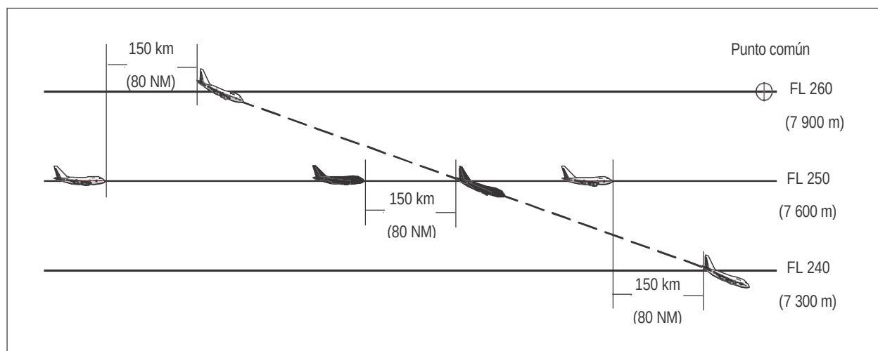
Figura 5-27B. Separación de 150 km (80 NM) basada en RNAV entre aeronaves que descienden y por la misma derrota [véase 5.4.2.5.5 c)]
