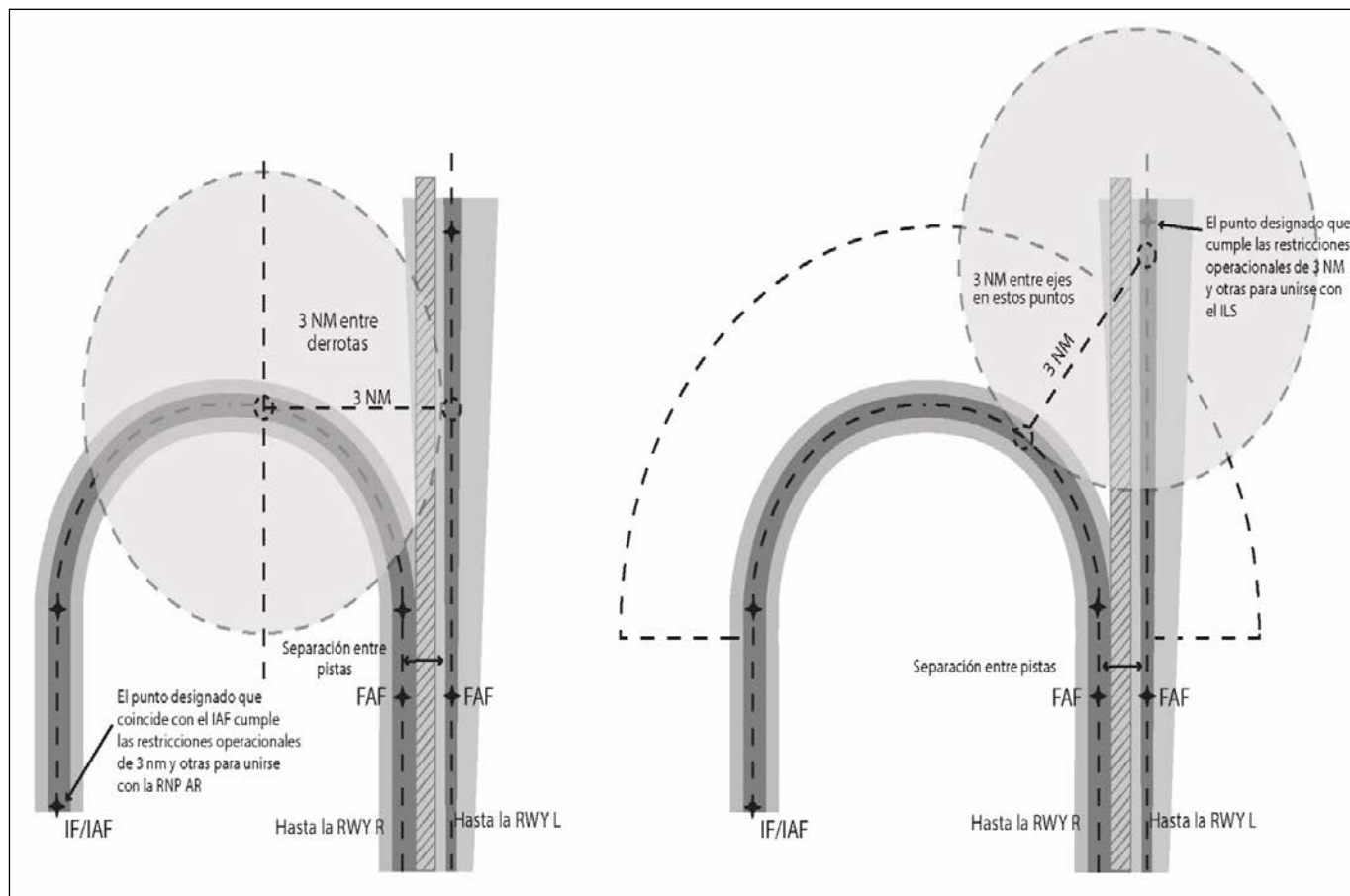
Figura 6-6. El concepto de ‘Establecida en la RNP AR APCH’ (Ejemplo de una aproximación RNP AR APCH/de precisión con una separación mínima de 3 NM)
