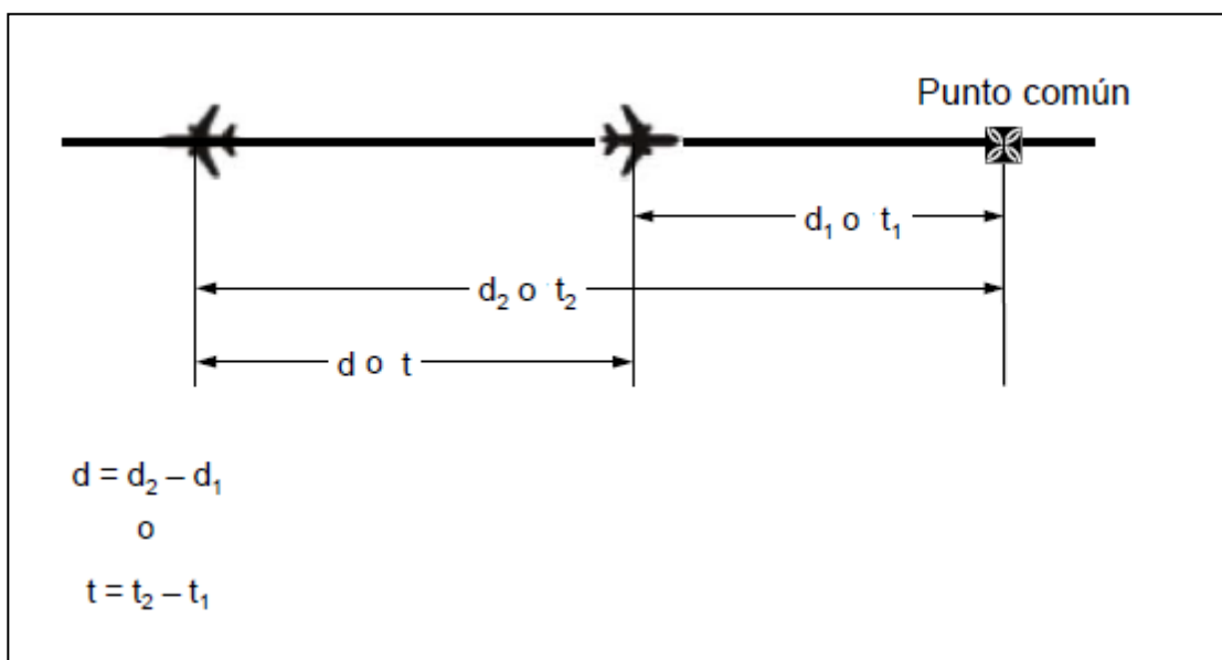
Figura 5-31. Cálculo de la distancia/tiempo longitudinal entre aeronaves — derrota idéntica, sentido opuesto [véase 5.4.2.9.5 a)]
