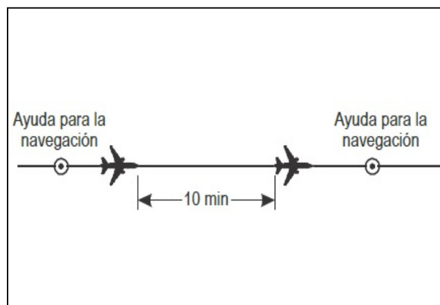
Figura 5-11. Separación de 10 minutos entre aeronaves por la misma derrota y el mismo nivel [véase 5.4.2.2.1.1 b)]
