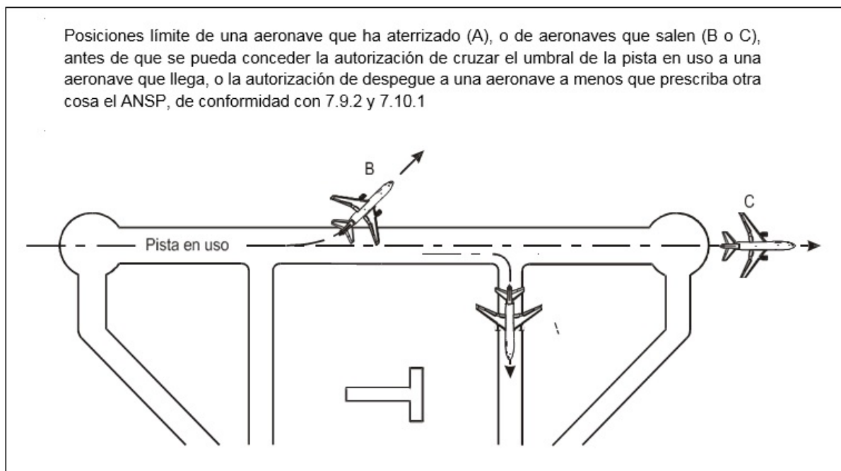
Figura 7-3. Separación entre aeronaves que llegan y salen (véanse 7.9.2 y 7.10.1)
