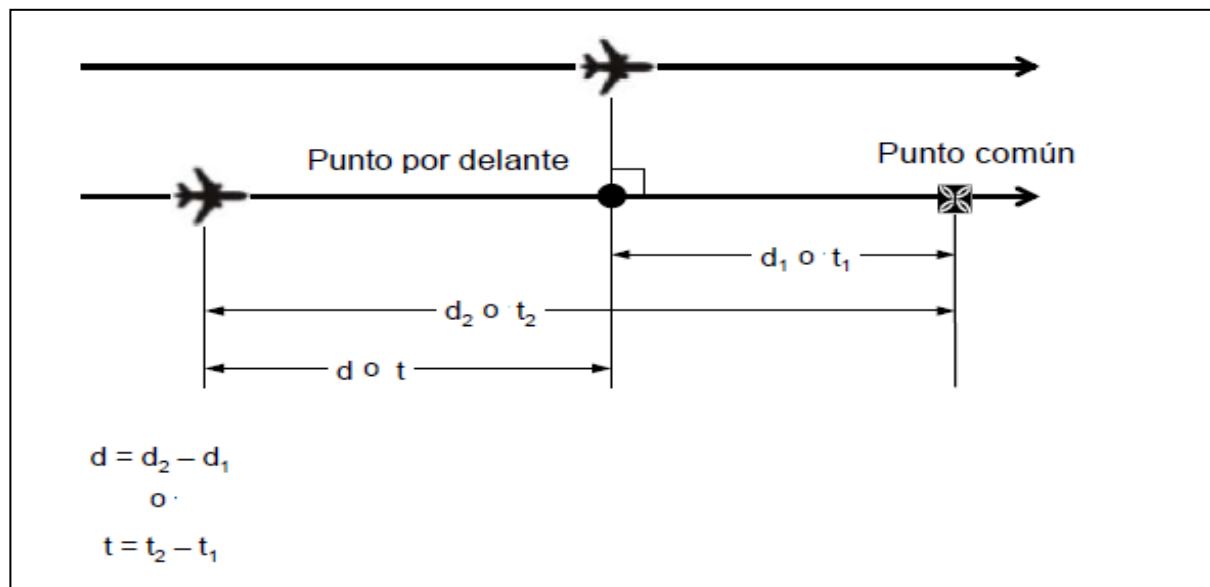
Figura 5-35. Cálculo de la distancia/tiempo longitudinal entre aeronaves — derrota paralelas [véase 5.4.2.9.5 c)]
