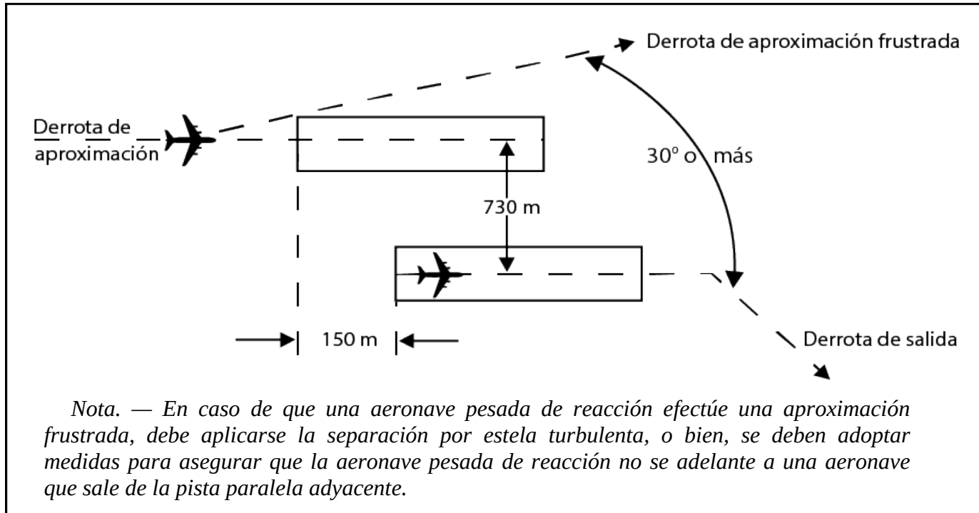
Figura 6-8. Operaciones paralelas segregadas cuando las pistas están escalonadas (véase 6.7.3.6.2)
