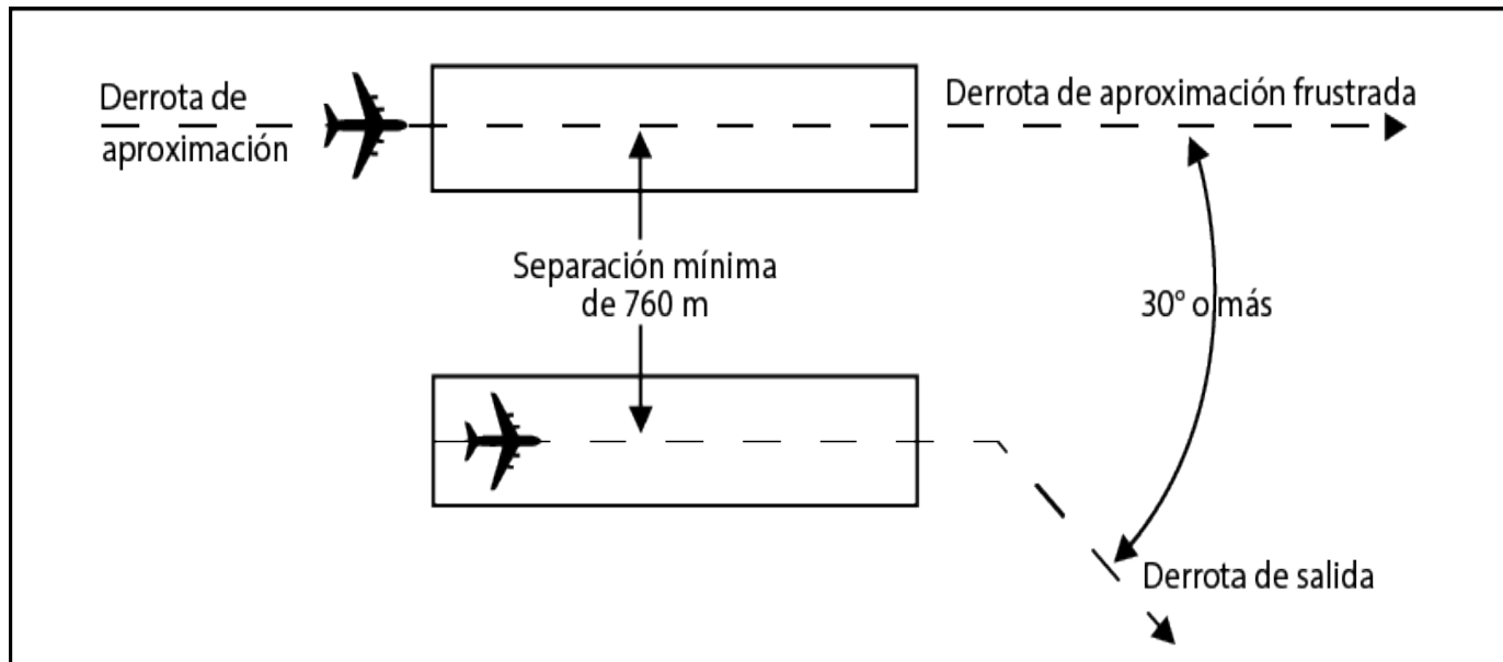
Figura 6-7. Operaciones paralelas segregadas [véase 6.7.3.6.1 b)]
