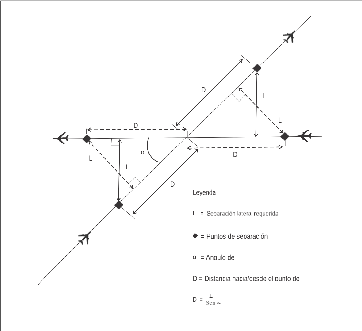
Figura 5-6. Puntos de separación lateral (véase 5.4.1.2.1.7) IF-2018-49512400-APN-DNINA#ANAC
