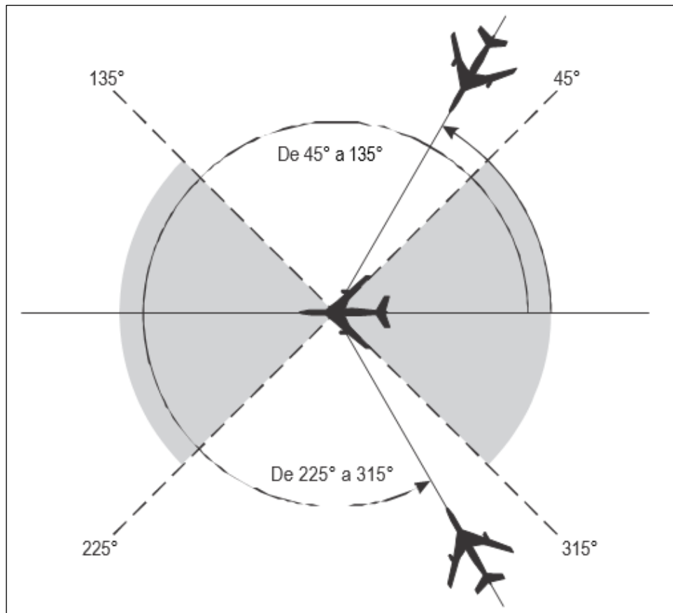
Figura 5-9. Aeronaves por derrotas que se cruzan [véase 5.4.2.1.5 c)]
